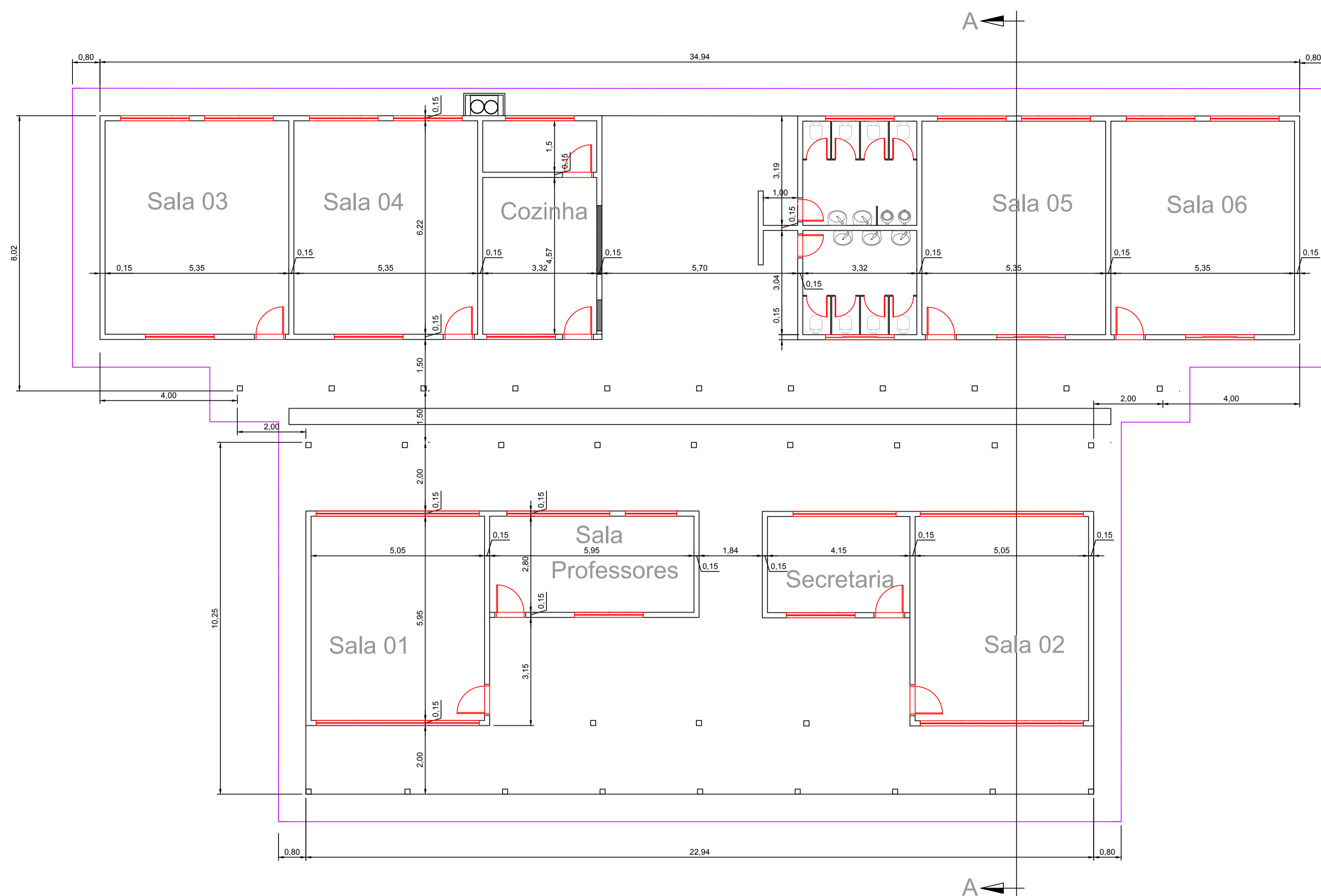
PLANTA BAIXA
